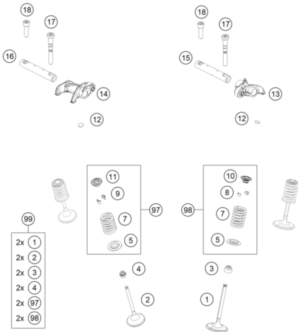
AUSLASS / EXHAUST
