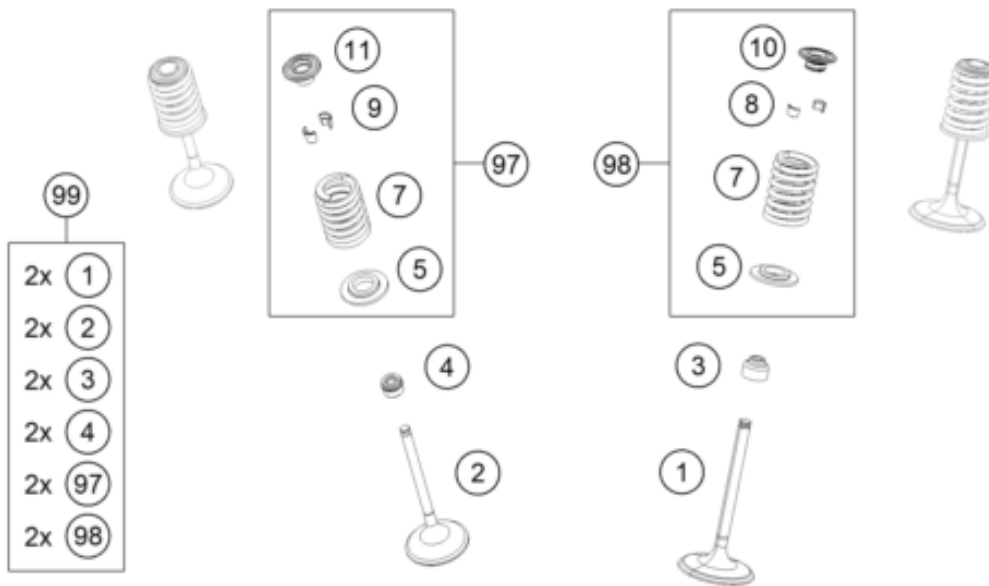
AUSLASS / EXHAUST
