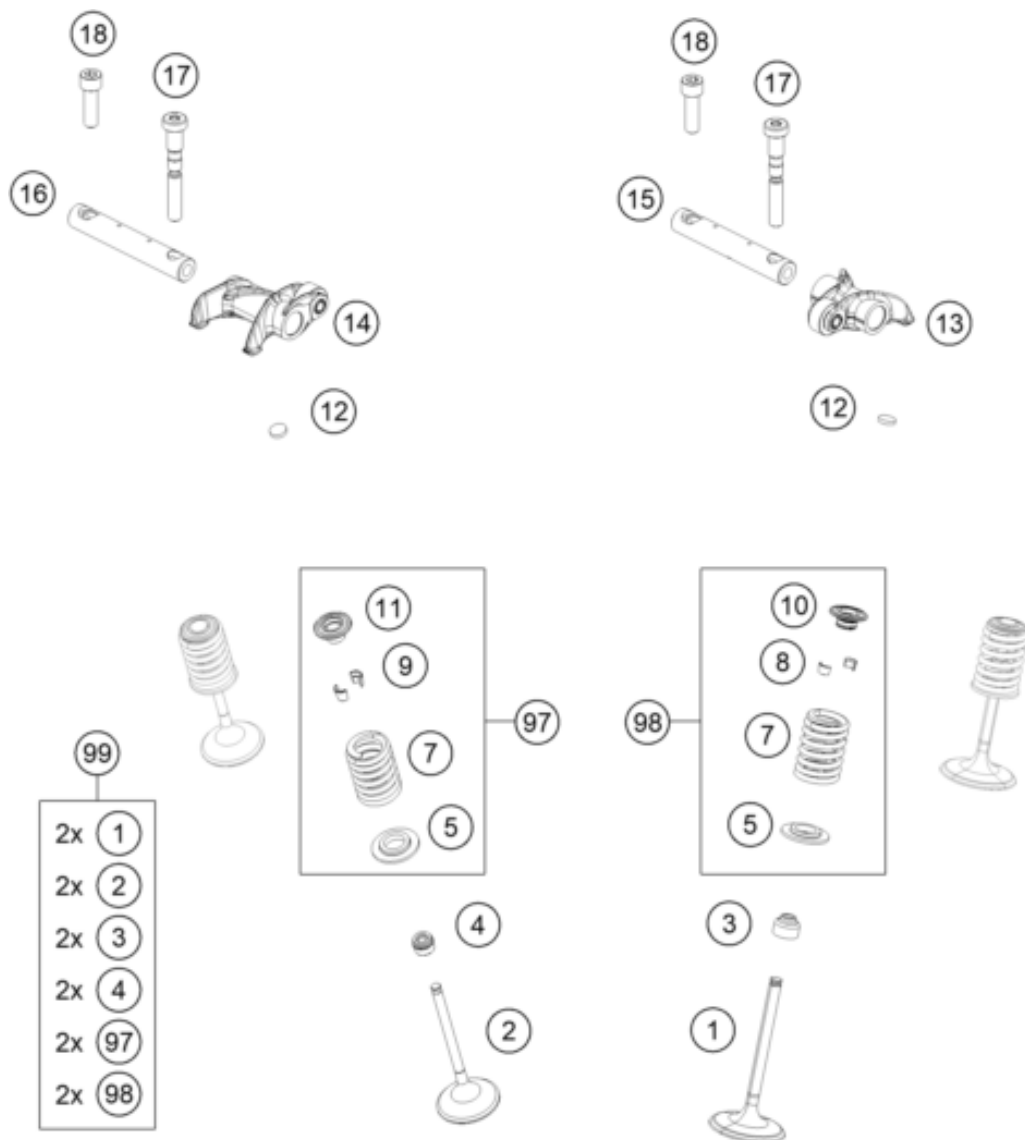
AUSLASS / EXHAUST
