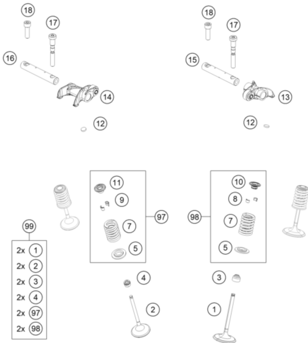
AUSLASS / EXHAUST
