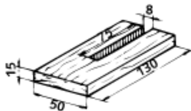
HOLZPLATTE - SELBSTGEFERTIGT WOODEN PLATE - HOME MADE
