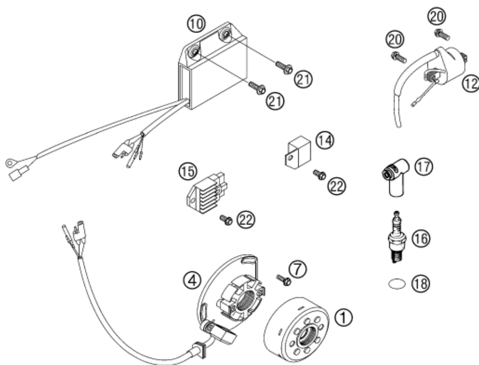
2K-1 (125 SX)
