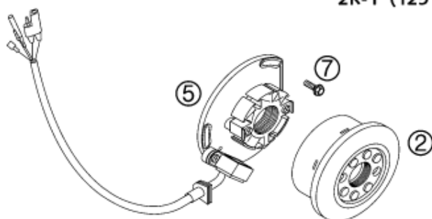
2K-2 (125-200 MXC/EXC-USA)
